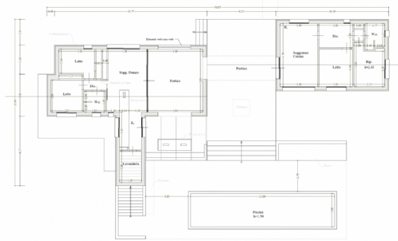
PIANTA PIANO TERRA (Modificato)
