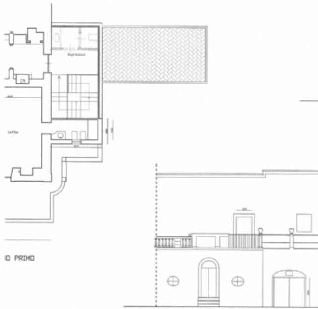
PROSPETTO LATERALE
